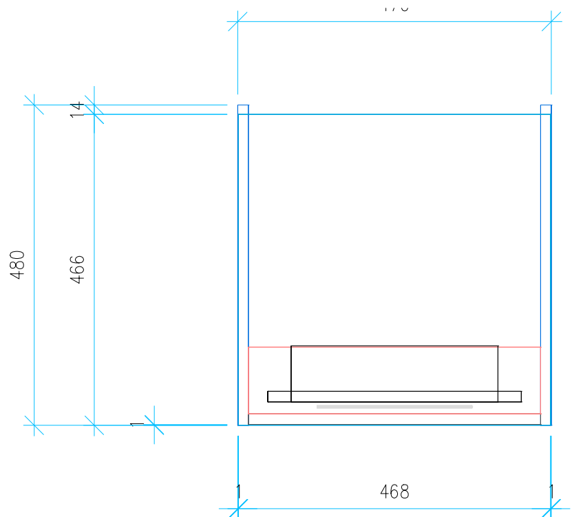
Ansicht 4 / Vorderansicht
